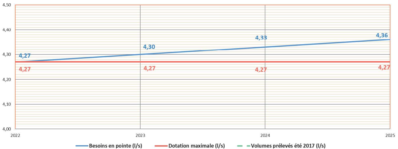
Équation 7: Evolution des besoins en pointe de 2022 à 2025 – MONS – Situation HIVER
